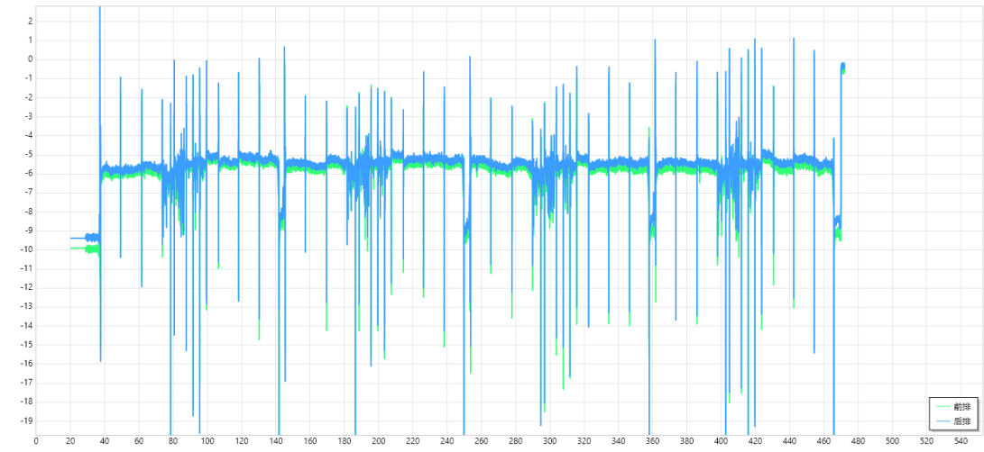
图 3 漏磁周向数据（横轴单位：米；纵轴单位：高斯）
