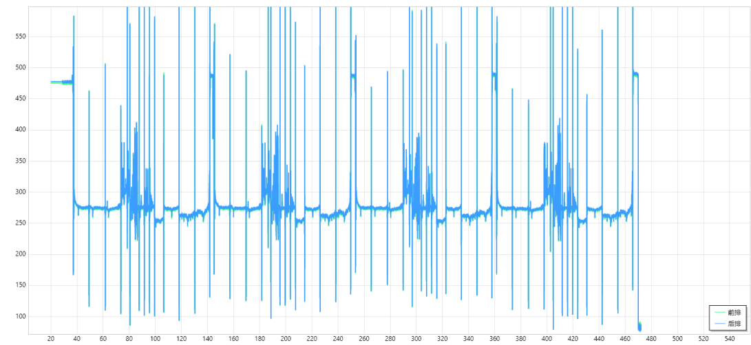
图 1 漏磁轴向数据（横轴单位：米；纵轴单位：高斯）
