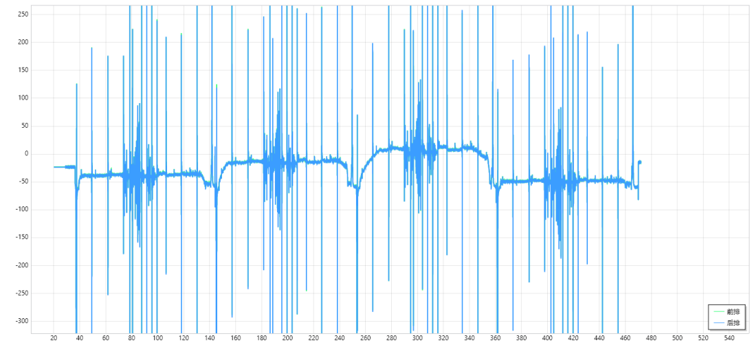
图 2 漏磁径向数据（横轴单位：米；纵轴单位：高斯）
